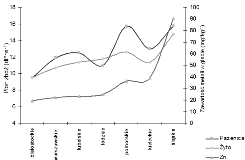
Rysunek 3. Plonowanie pszenicy i żyta w badanych województwach Polski przedwojennej na tle zawartości cynku (Zn) w glebach tych województw Źródło: Opracowanie własne.
